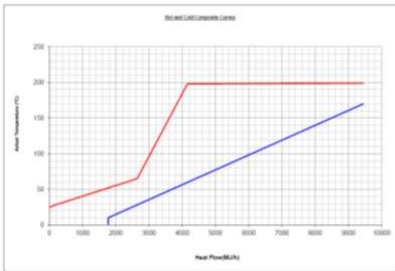
Diagramme température/enthalpie du séchoir avant insertion de pompe à chaleur
